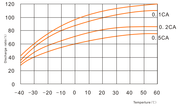
Temperture and discharge capacity / Température et capacité de décharge
