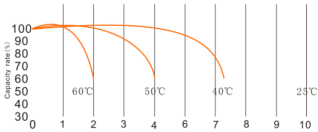
Temperture and float service life / Température et durée de vie
